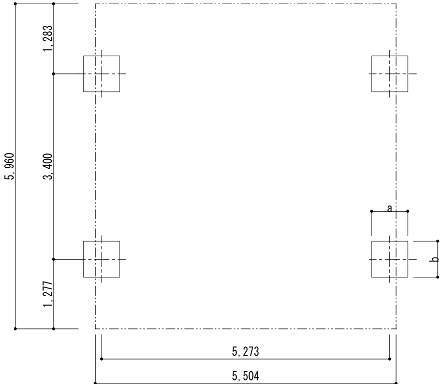
■ 基礎配置図
